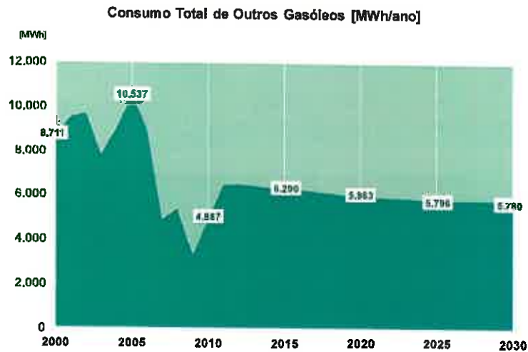
Figura 30 - Consumo Total de Outros Gasóleos [MWh/ano]
