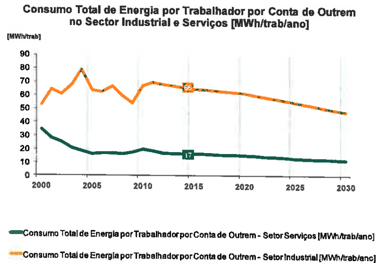
Figura 37 - Consumo Total de Energia por Trabalhador por Conta de Outrem no Sector Industrial e Serviços [MWh/trab/ano]
