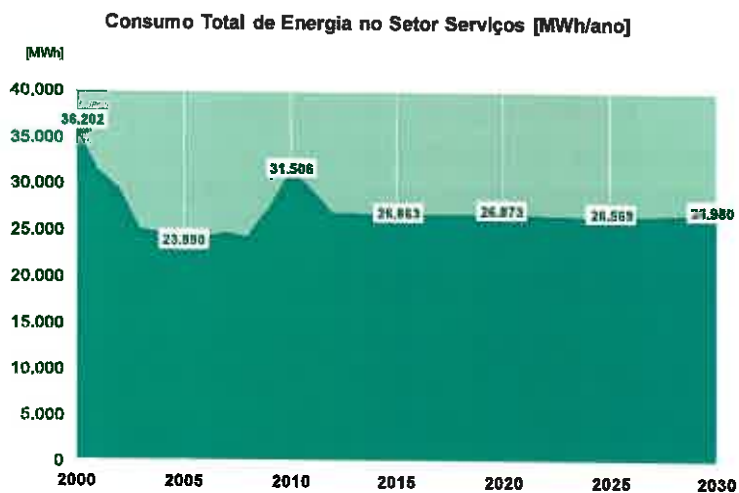
Figura 13 - Consumo Total de Energia no Setor Serviços [MWh/ano]
