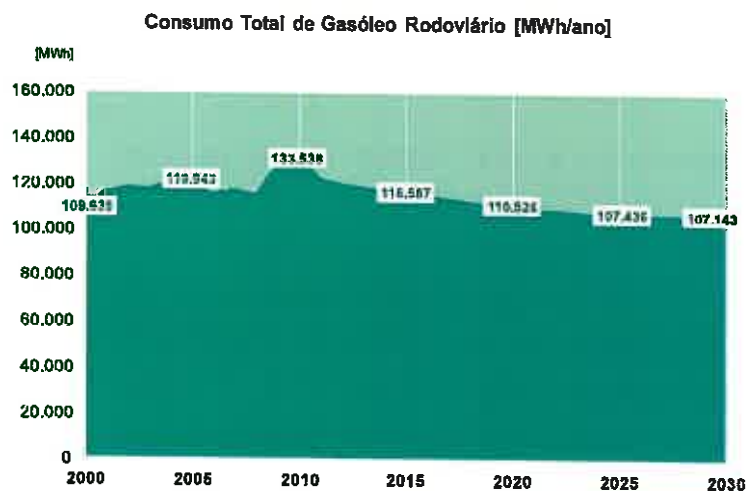
Figura 29 - Total de Gasóleo Rodoviário [MWh/ano]
